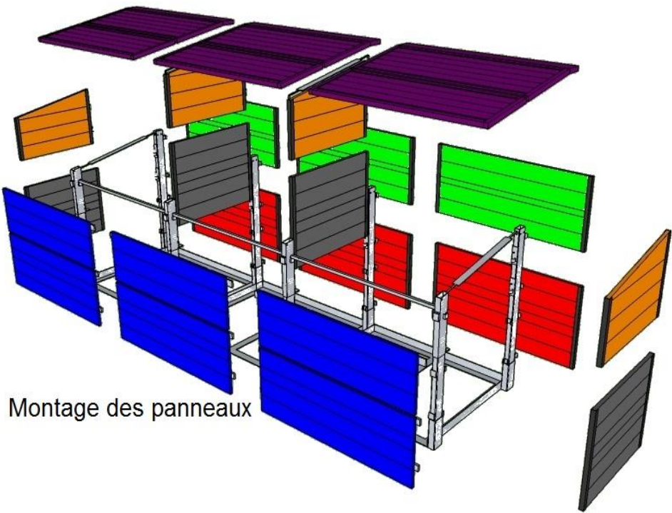
Vue éclatée
